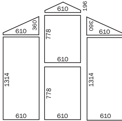
Frontwand
