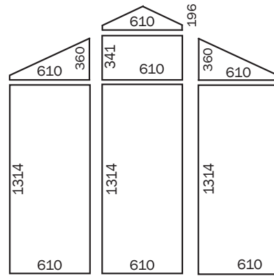
Rückwand
