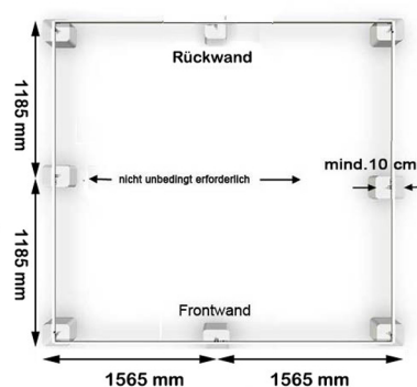
Bemaßung: Aussenkanten Punktfundament
