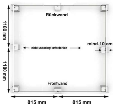
Bemaßung: Aussenkanten Punktfundament
